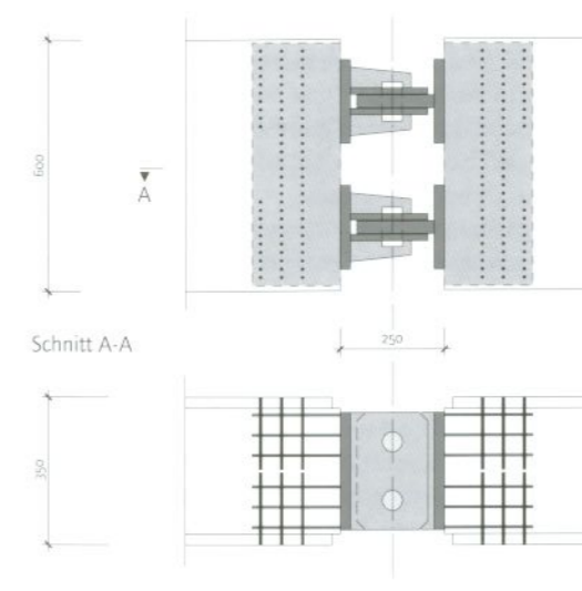
Abb. 3: Verbindung am Untergurt
